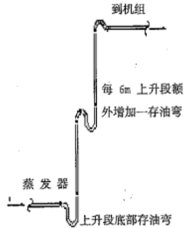
图3 机组高于蒸发器的情况
