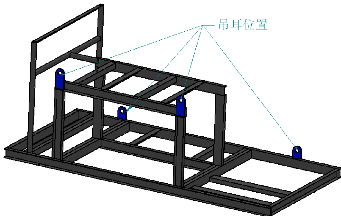
图 2 用于吊装的 4 只吊耳在机架上的位置
