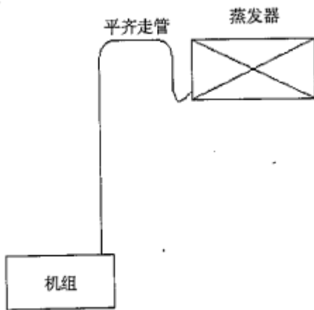
图5 蒸发器高于机组的情况
